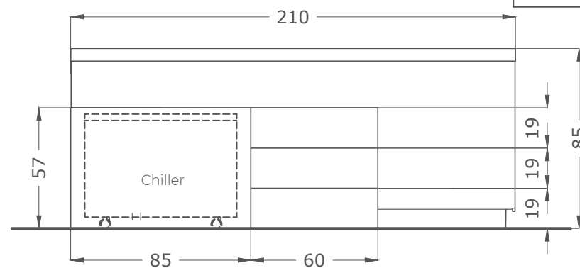
Prospetto frontale
