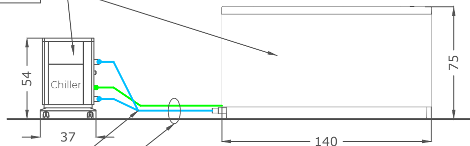
Prospetto frontale
