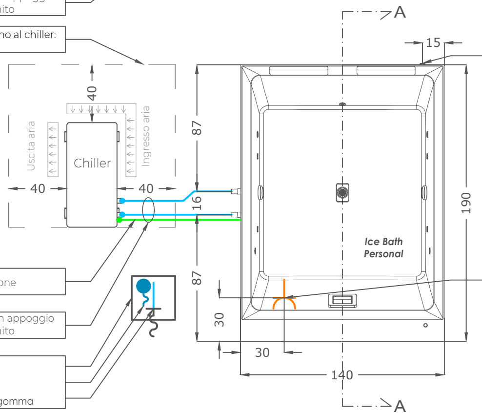
Pianta
