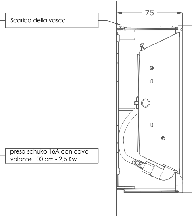
Prospetto laterale
